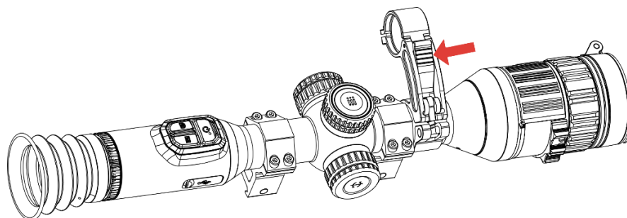
Obrázek 2-11 Uzamčení páčky
