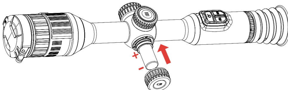
Obrázek 2-3 Vložení baterie
