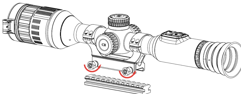
Obrázek 2-8 Uvolnění šroubů
